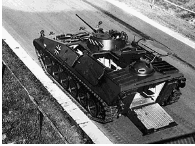
RU 361 von 1966 – die Prototypen des SPz-neu wachsen: hier das erste Fahrzeug mit sechs Laufrollen und erstmals dabei: die Hecklafette
